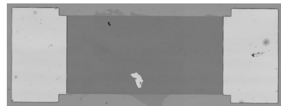
Powiększenie mikroskopowe badanej struktury – tranzystora FET z widocznymi kontaktami źródła i drenu oraz jednoatomową warstwą grafenu między nimi, stanowiącą warstwę gazoczułą
