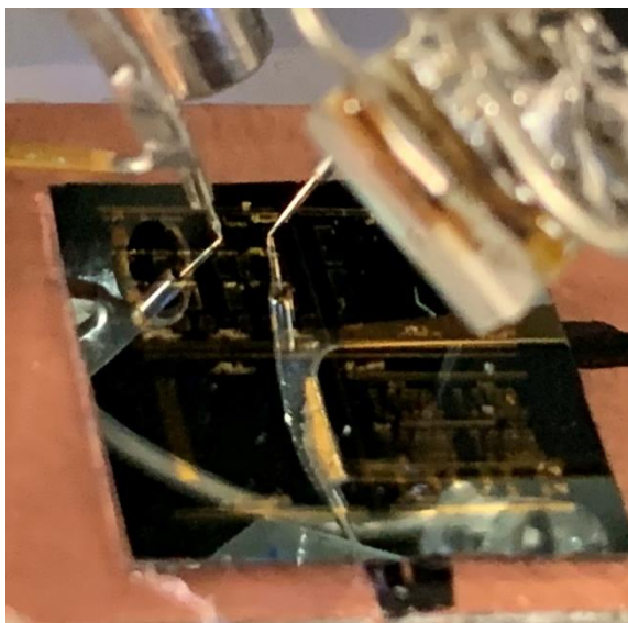
Badane struktury, dołączane do układu pomiarowego tytanowymi igłami
